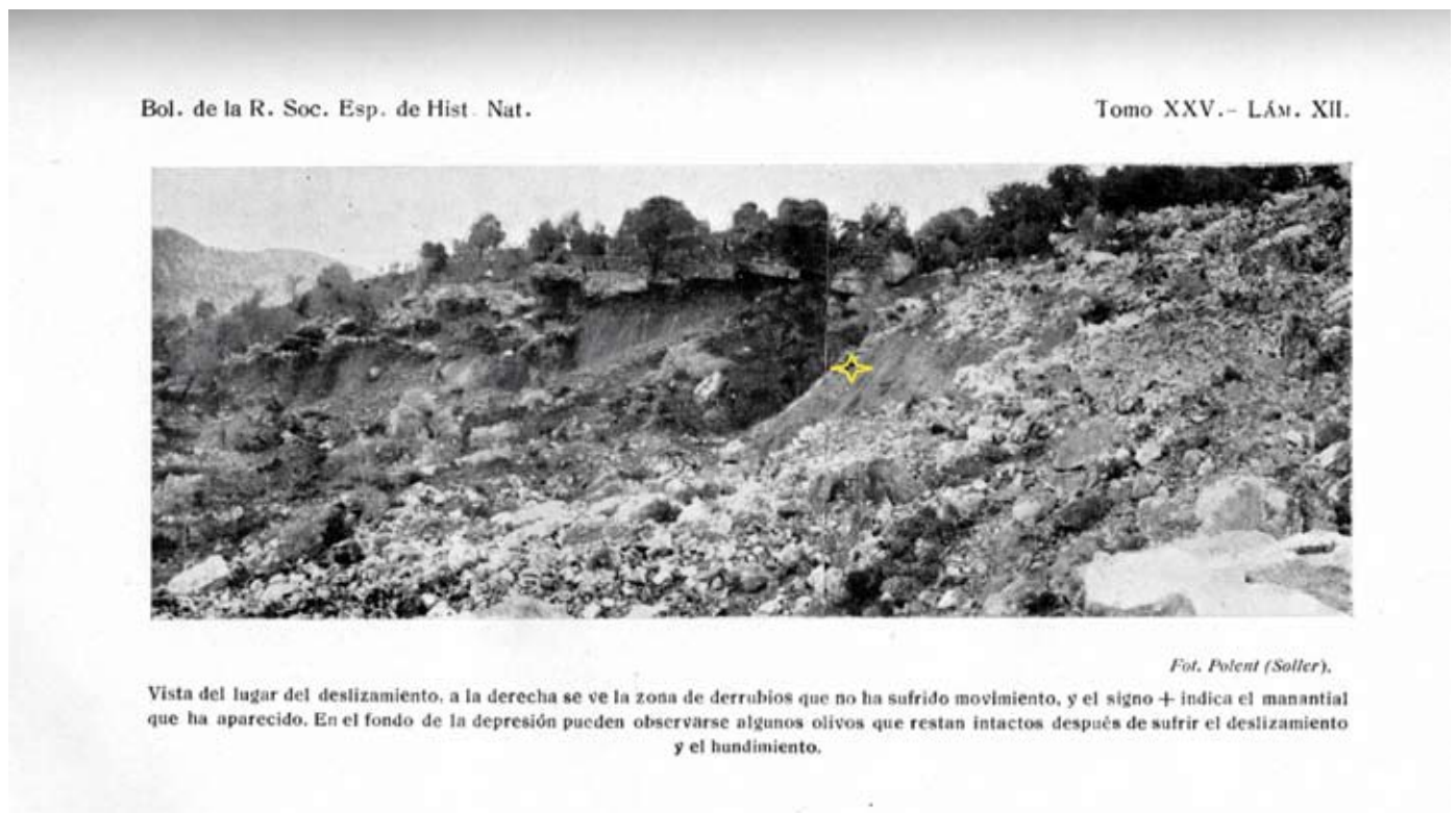
Figura 8. Reproducción de la fotografía realizada por Darder al deslizamiento en pleno movimiento. Nótese las observaciones realizadas por el autor en el pie de la figura donde refiere la aparición de un manantial en el punto señalado con una cruz (resaltado en amarillo).
