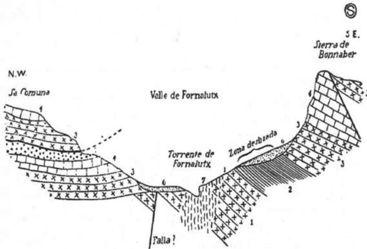
Fig. 1.—Corte geológico del valle de Fornalutx.
