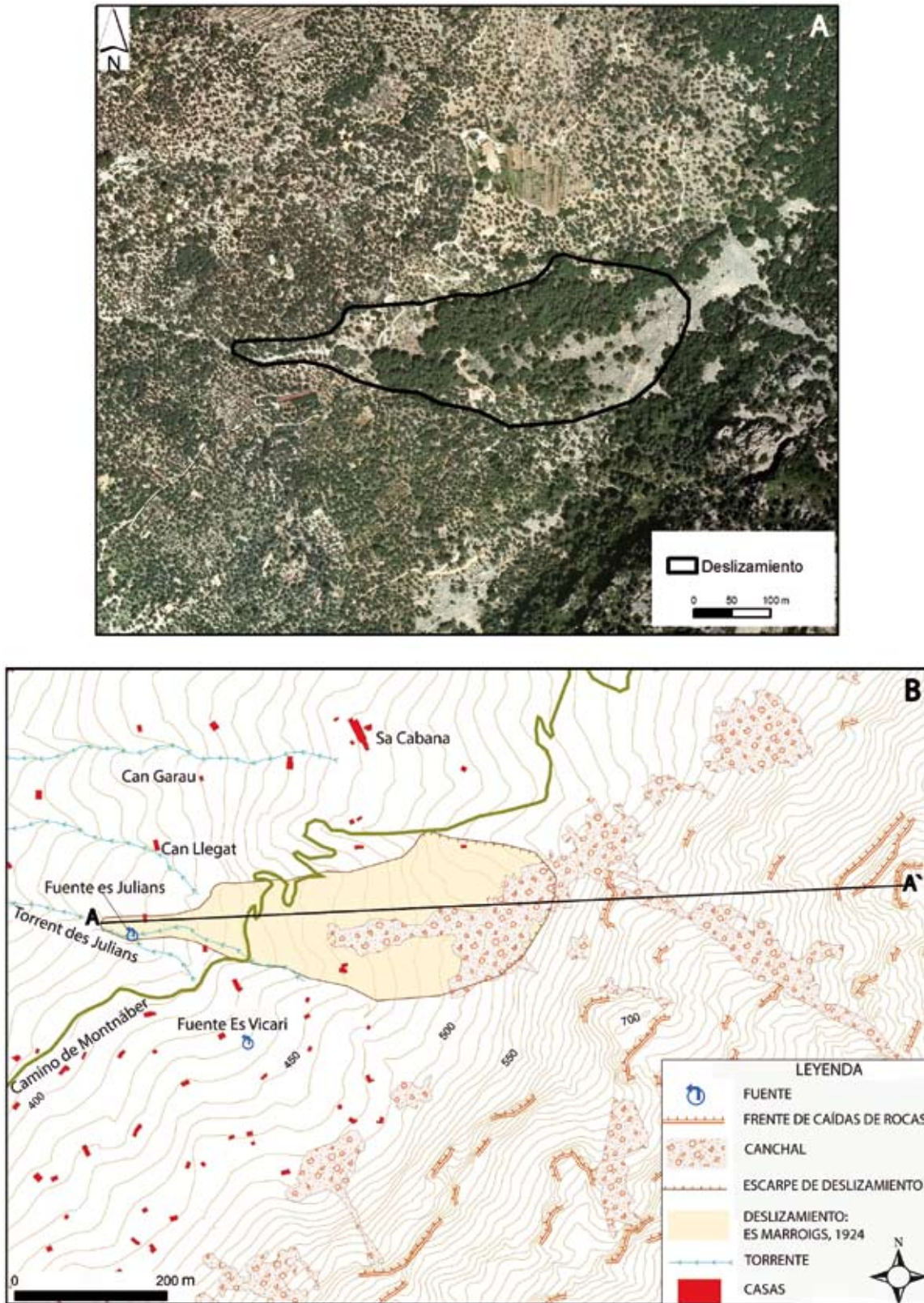
Figura 6. A) Fotografía aérea de la zona donde se observa con claridad la invasión de los bloques procedentes del canchal sobre el deslizamiento. B) cartografía del deslizamiento sobre la base topográfica. Se ubica el trazado del corte geológico de la Fig. 7. Figure 6. A) Aerial photograph where the rock blocks from the scree invading the landslide can be observed. B) Topographical map of the landslide. The cross section represented in Figure 7 is shown.
