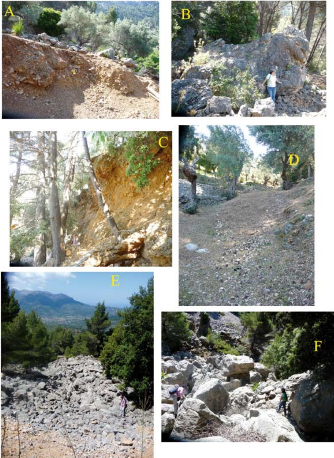
Figura 5. Observaciones en campo del deslizamiento. A: Masa deslizada con una granuloclasificación inversa; B: Bloques de gran tamaño procedentes del canchal con signos de arrastre; C: Escarpe lateral del deslizamiento en su extremo norte, poniendo al descubierto las brechas cementadas del Pleistoceno D: Límite lateral del flujo de derrubios; E: Lengua de bloques procedentes del canchal invadiendo el deslizamiento; F: Cabecera del deslizamiento hundida e invadida por los bloques del canchal.
